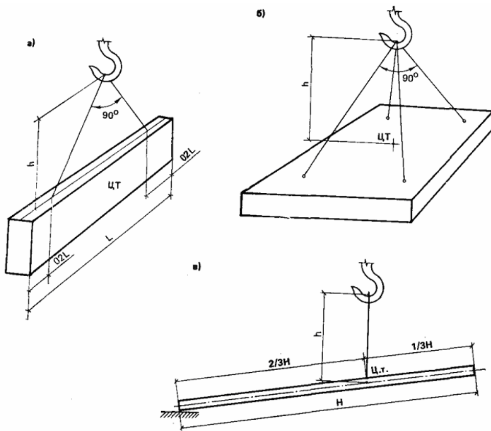
Рис. 4. Схема расположения точек строповки монтируемых конструкций
