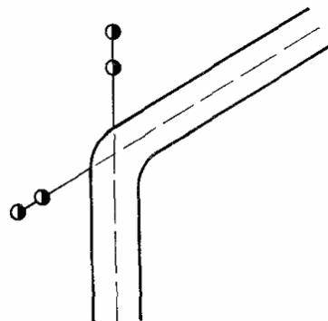
Рис. 10. Схема закрепления главных разбивочных осей углов поворота линейных сооружений
