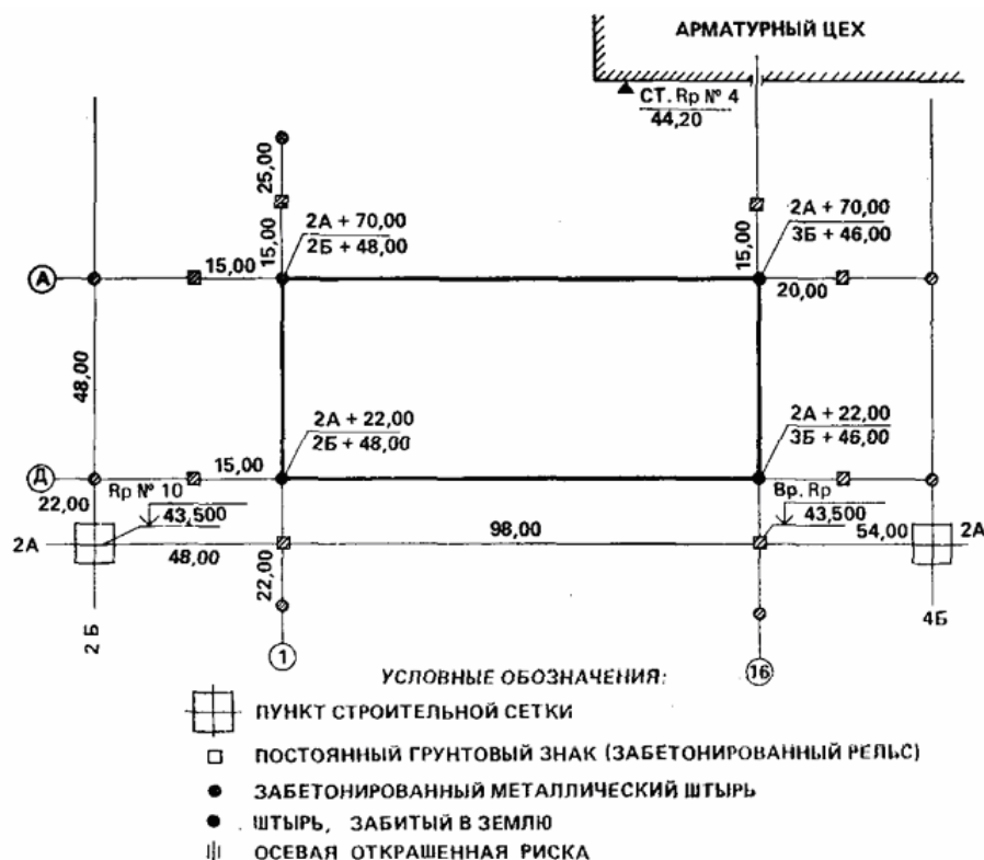
Рис. 14. Схема закрепления и привязки основных осей здания
