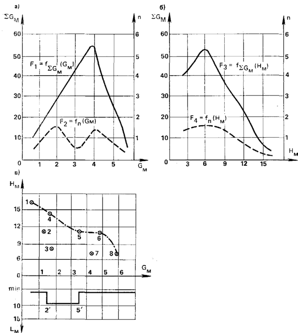
Рис. 2. Графики распределения характеристик монтажных элементов
