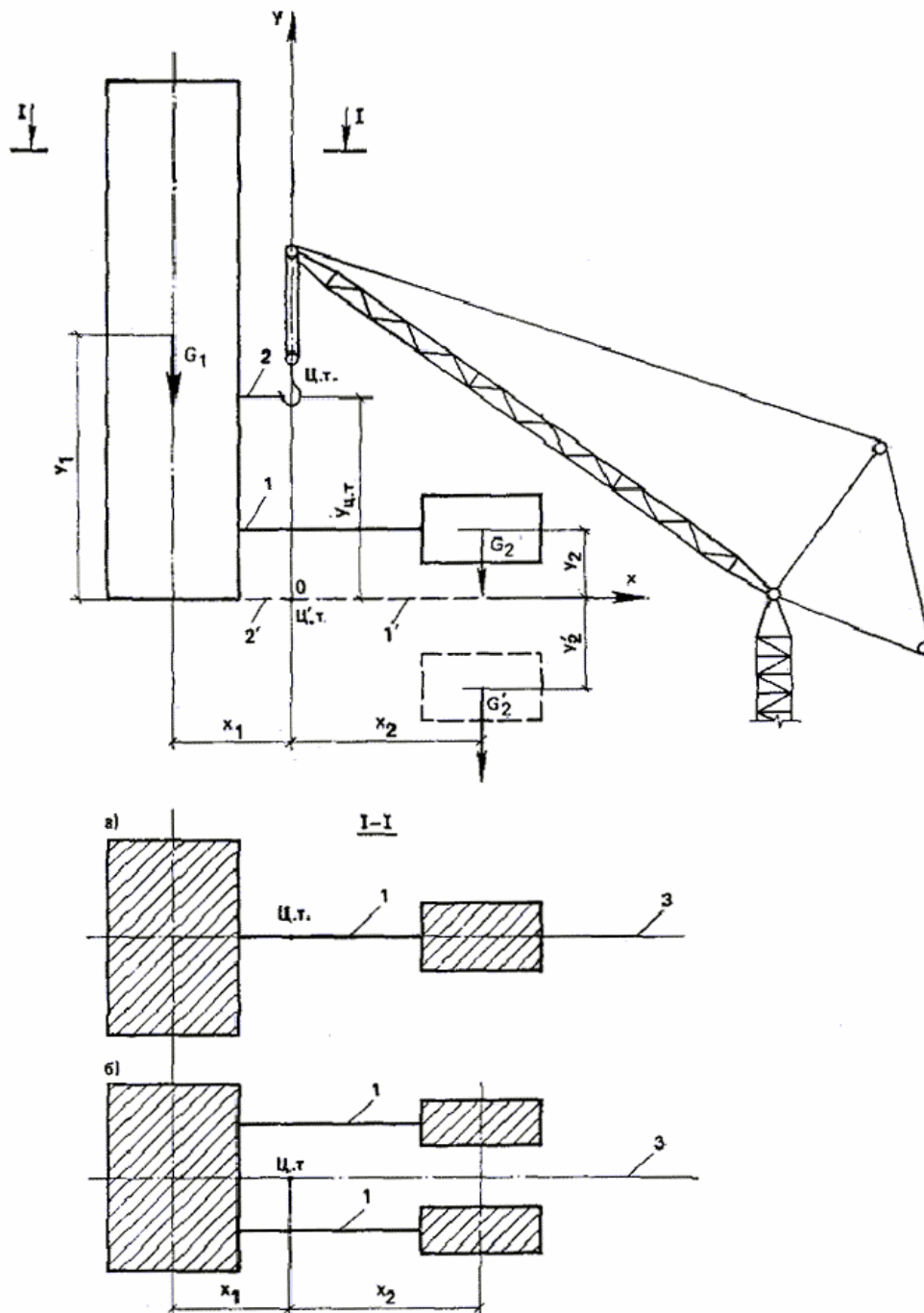
Рис. 5. Схема для определения координат центра тяжести строповочного узла, расположенного ниже центра тяжести монтируемой конструкции при размещении дополнительного груза с одной (а) и с двух (б) сторон стрелы
