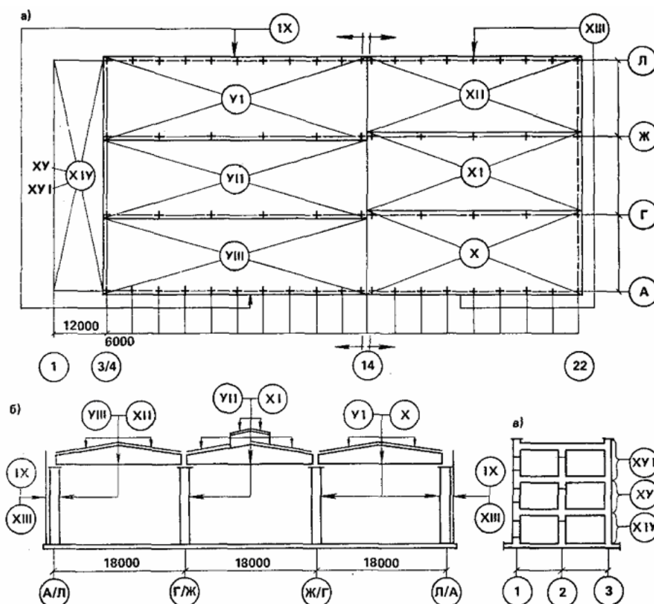
Рис. 13. Схема образования технологических комплексов при возведении одноэтажного здания (пример)
