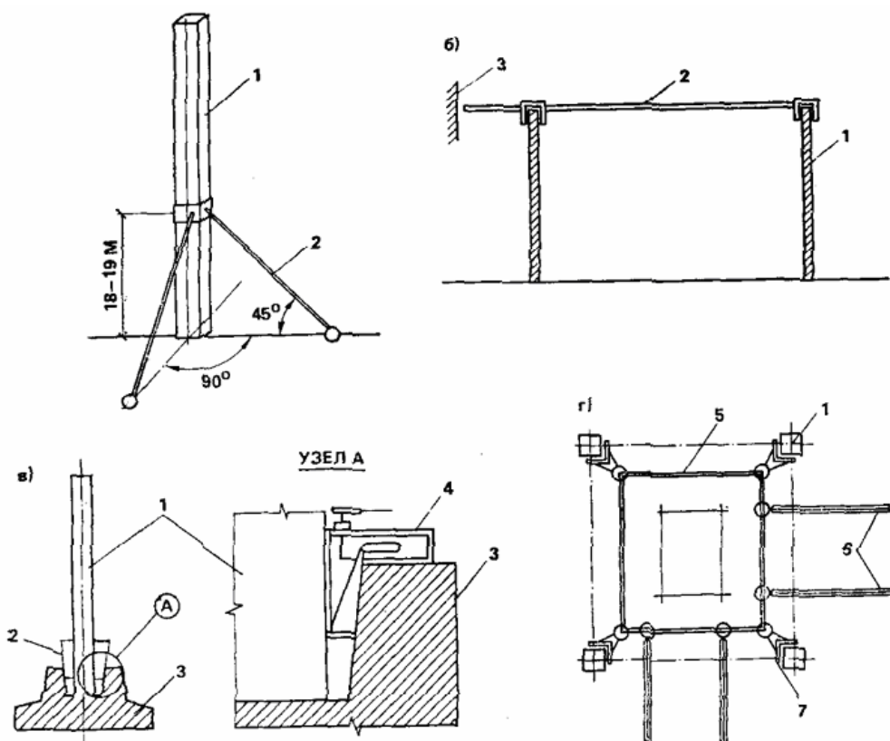
Рис. 7. Удерживающие приспособления
