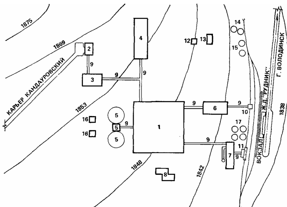
Рис. 6. Ситуационный план строительства обогатительной фабрики
