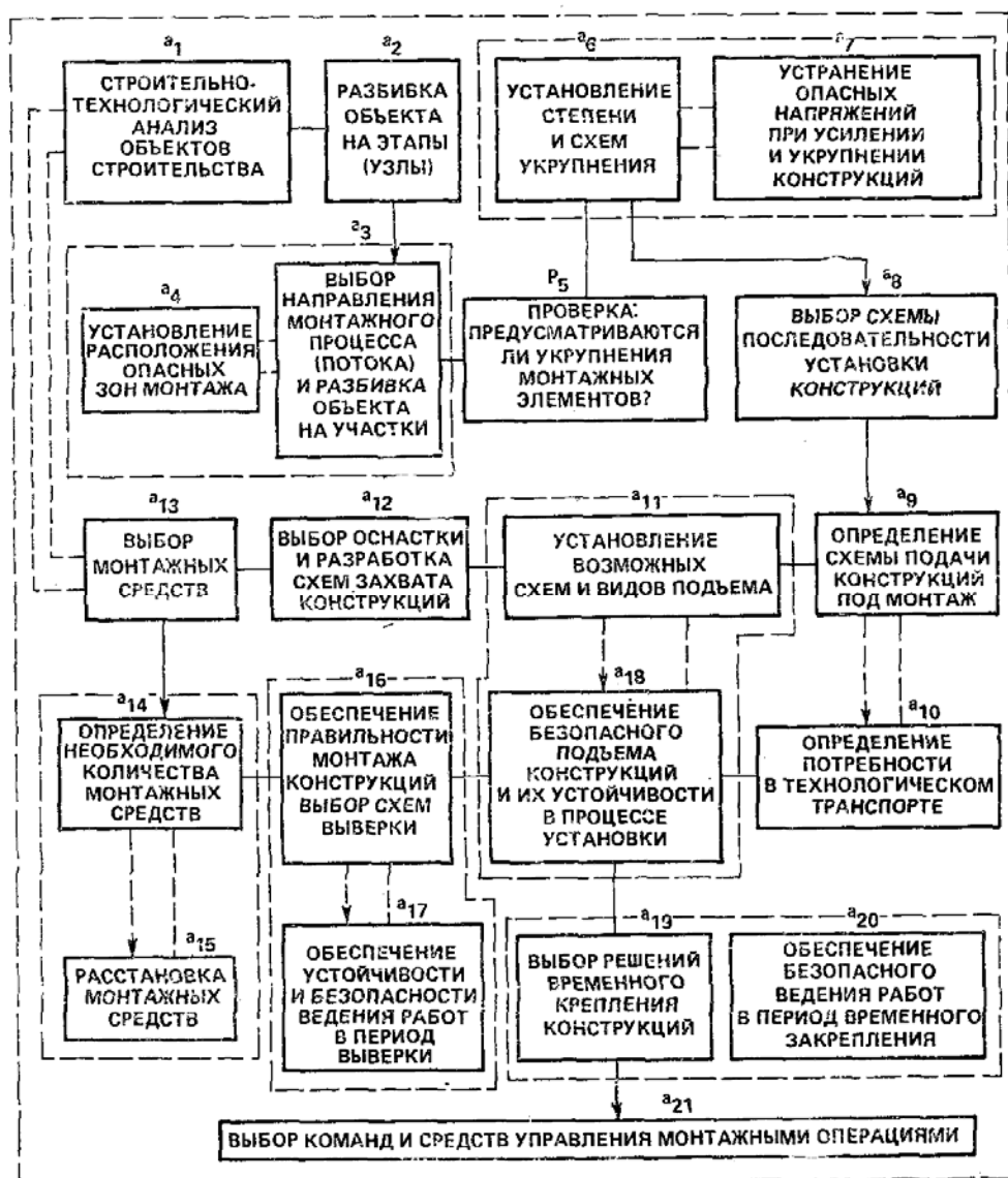
Рис. 1. Схема последовательности разработки вариантов методов монтажа
