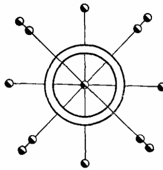
Рис. 8. Схема закрепления главных разбивочных осей сооружений башенного типа
